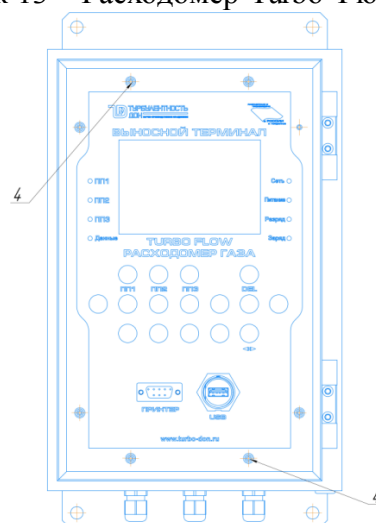
Рисунок 15 – Выносной терминал в металлическом корпусе (VTM)
