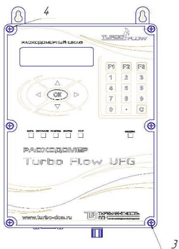
Рисунок 12 – Расходомерный шкаф
