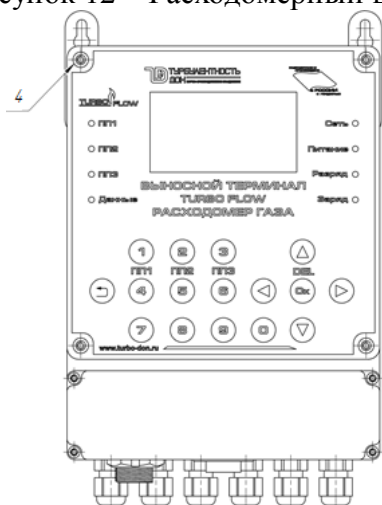
Рисунок 14 – Выносной терминал (VT)
