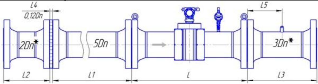
Рисунок Д.14 – Монтаж расходомера со струевыпрямителем со вставкой 2Dn класса точности В (1,0 % - 1,0 %) для исполнения корпуса V по стандарту ASME B16.5-2003
