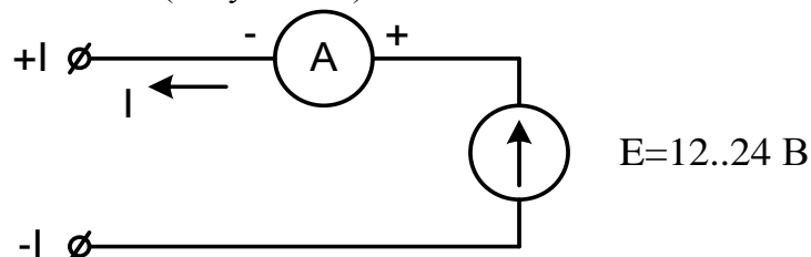
Рисунок 4.4 – Схема подключения приборов для проверки токового выхода
