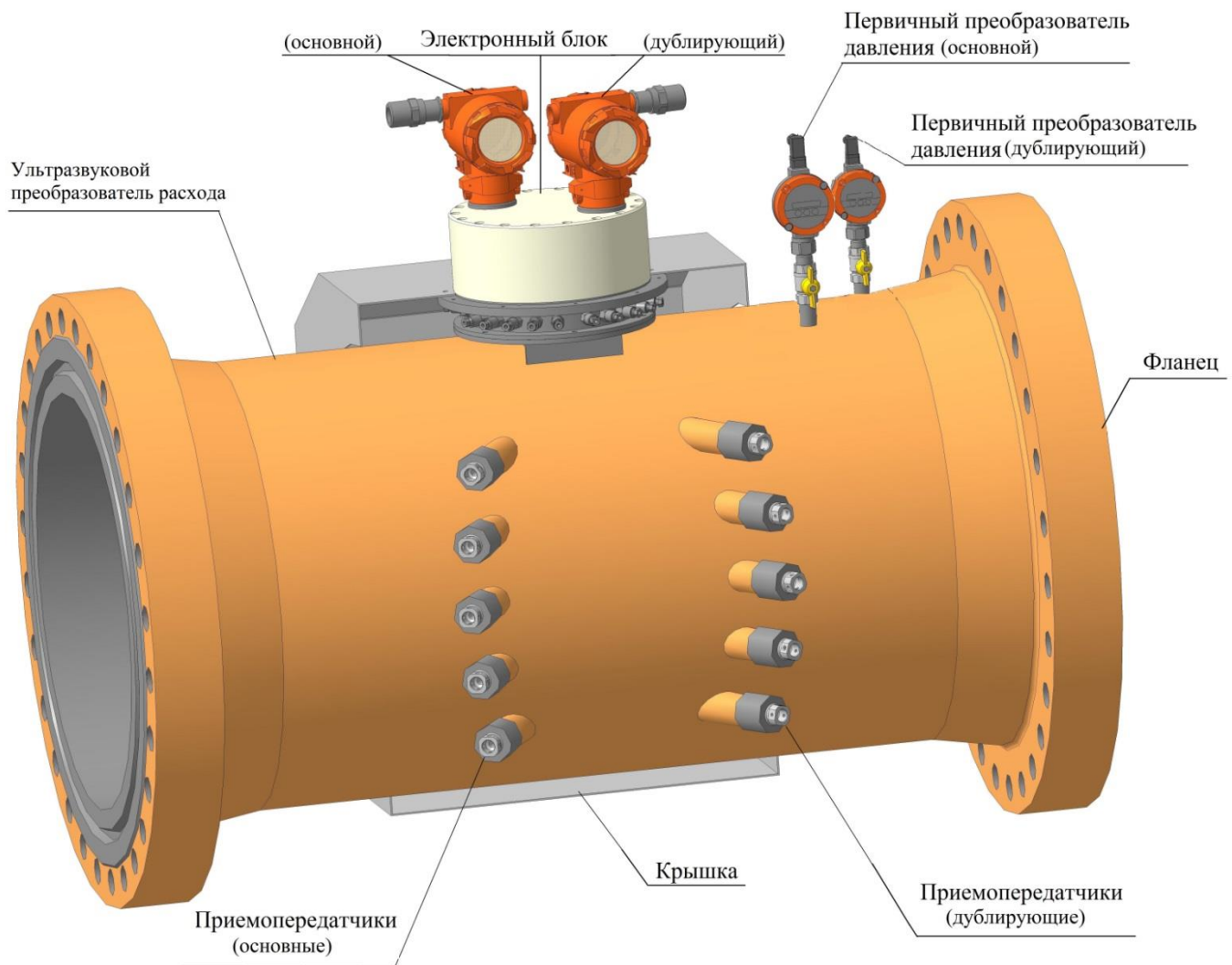
Рисунок Б.6 - Расходомер - счетчик газа ультразвуковой исполнения с дублированием
