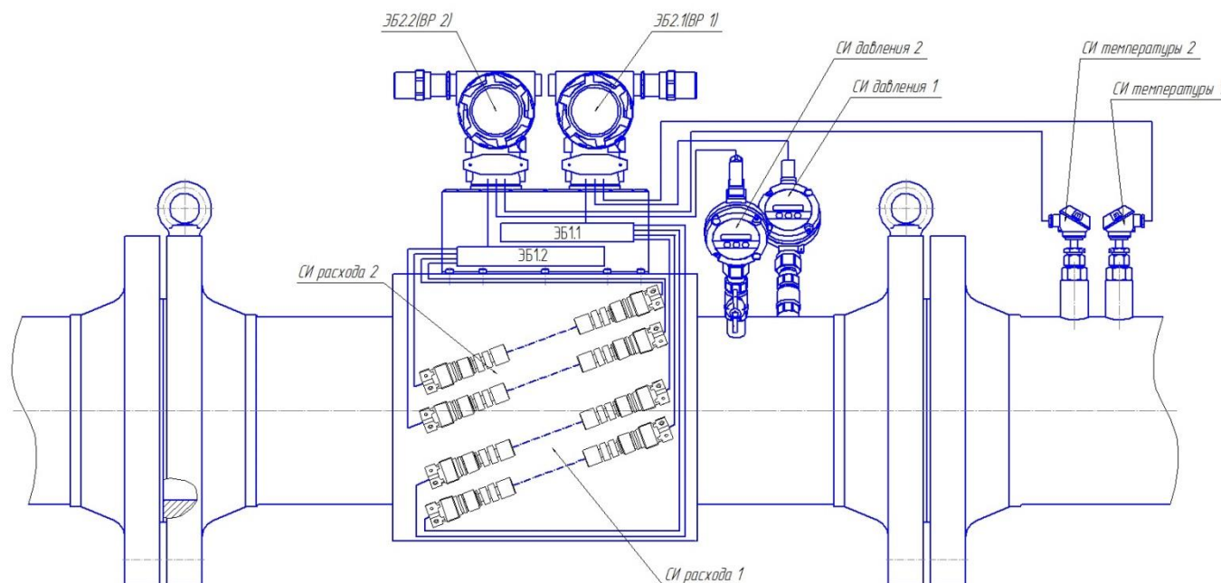
Рисунок 2.63 – Структурная схема дублирования вычислительных устройств (полное дублирование)
