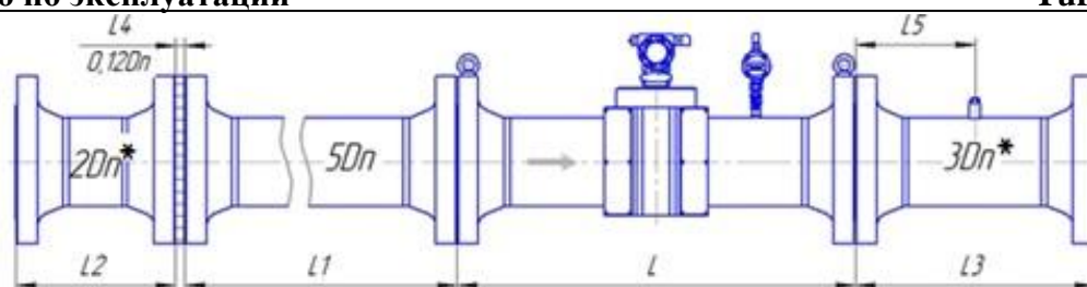
Рисунок Д.12 – Монтаж расходомера со струевыпрямителем укороченной длины со вставкой 2 Dn классов точности А (0,5 %-0,3 %) и Б (0,5 %-0,5 %) для исполнения корпуса V по стандарту ASME B16.5-2003
