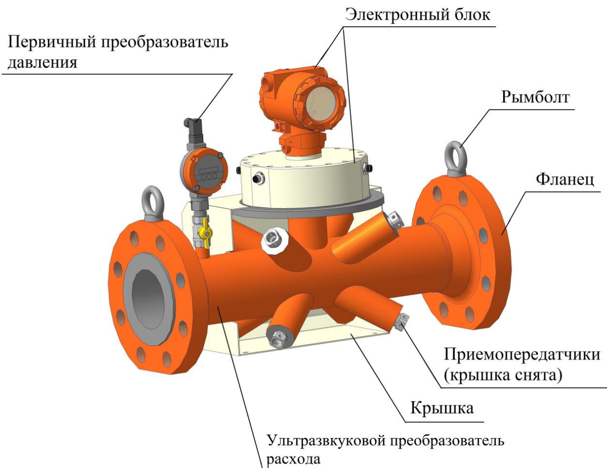
Рисунок Б.4 – Расходомер - счетчик газа ультразвуковой исполнение корпуса V, VR
