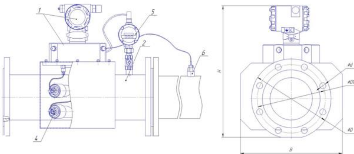
Рисунок Б.4 – Расходомер - счетчик газа ультразвуковой исполнение корпуса V, VR
