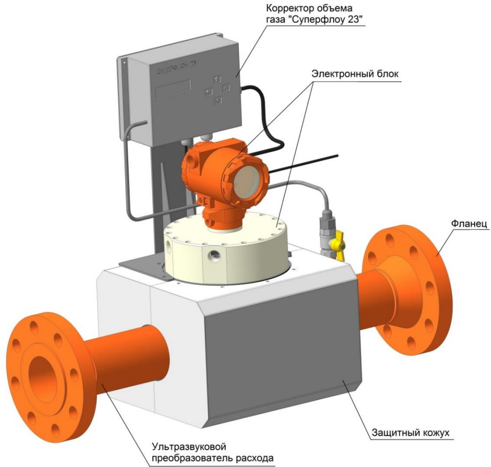
Рисунок Б.7 – Расходомер - счетчик газа ультразвуковой исполнение корпуса V, VR с внешним ВР Суперфлоу-23 (исполнение С4)
