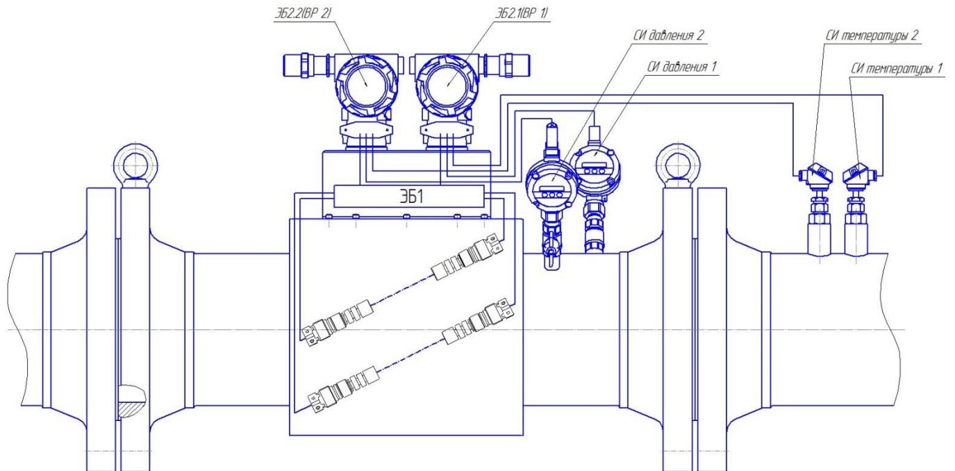
Рисунок 2.65 – Структурная схема дублирования вычислительных устройств (частичное дублирование)
