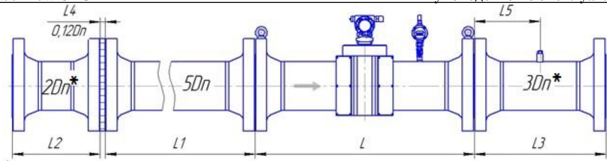
Рисунок Д.5 – Монтаж расходомера со струевыпрямителем со вставкой 2Dn класса точности В (1,0 % - 1,0 %) для исполнения корпуса V и С с типом присоединительных фланцев по ГОСТ 33259
