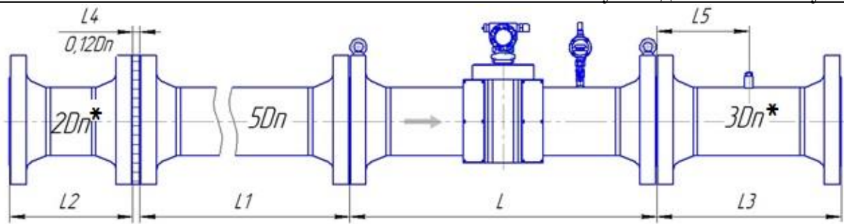
Рисунок Д.3 – Монтаж расходомера со струевыпрямителем укороченной длины со вставкой 2Dn классов точности А (0,5 % - 0,3 %) и Б (0,5 % - 0,5 %) для исполнения корпуса V и С с типом присоединительных фланцев по ГОСТ 33259
